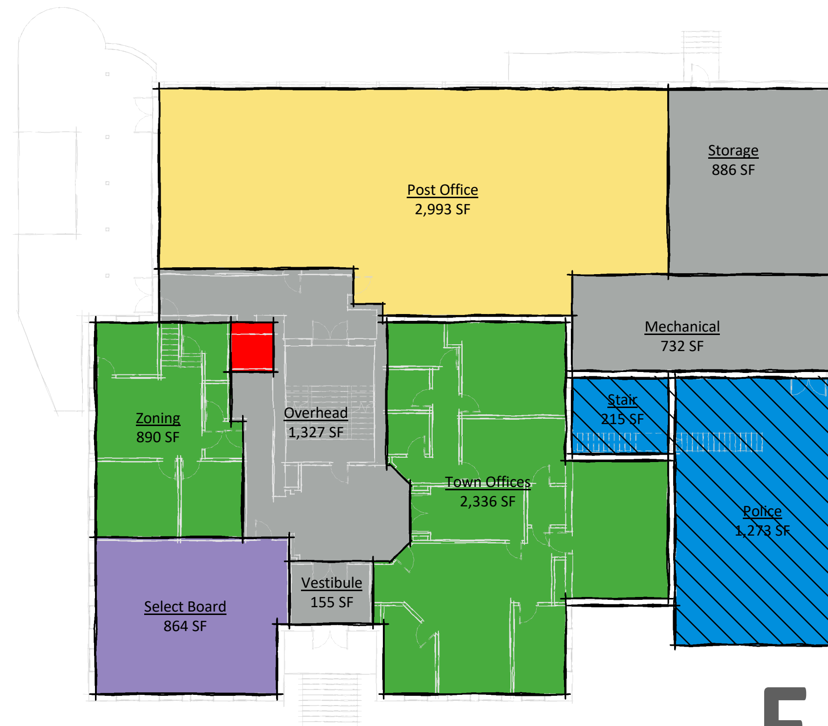
6 E - Level 2 SCALE: 1/16" = 1'-0"
