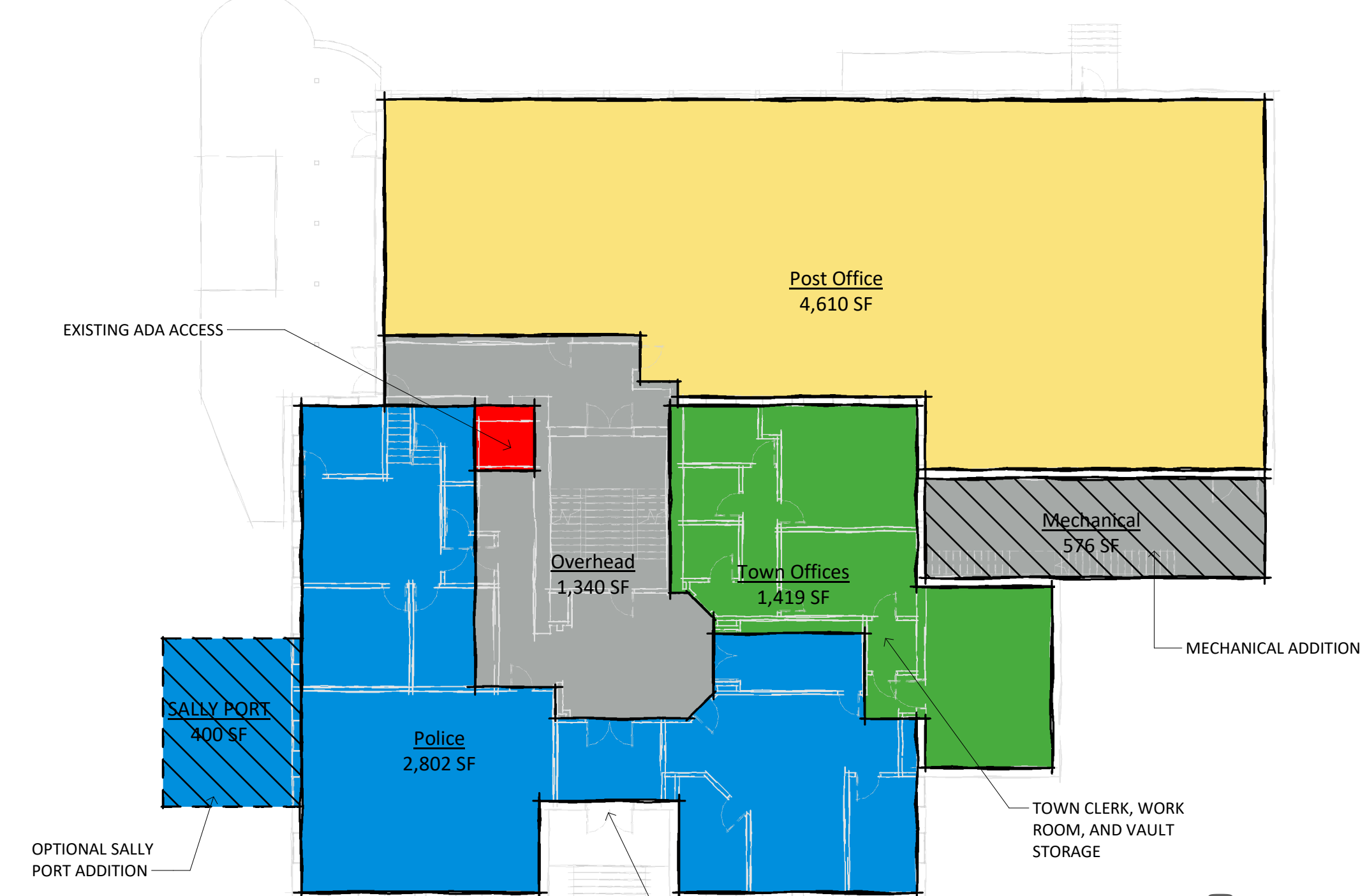
3 A - Level 2 SCALE: 1/16" = 1'-0"
